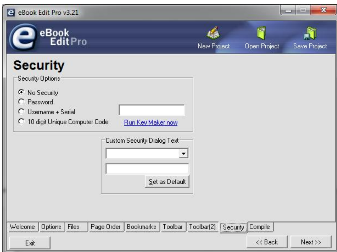
Рис. 3. Окно безопасности
